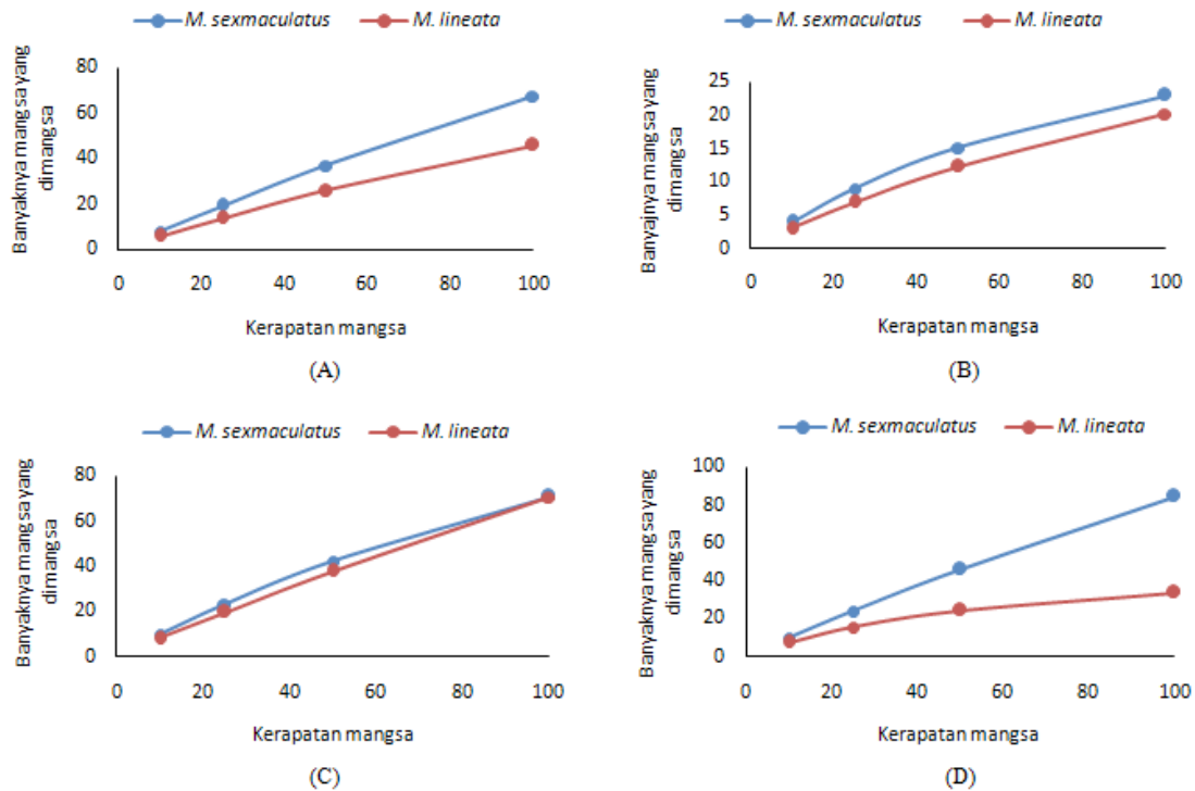
Gambar 1. Tipe tanggap fungsional Menochilus sexmaculatus dan Micraspis lineata terhadap nimfa Bemisia tabaci (A), pupa B. tabaci (B), Nimfa Myzus persicae (C), dan imago M. persicae (D).
